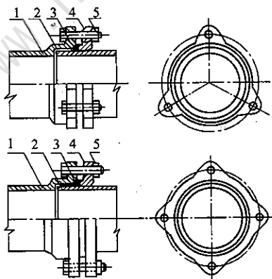
图2 铸铁管法兰机械式接口连接示意图
